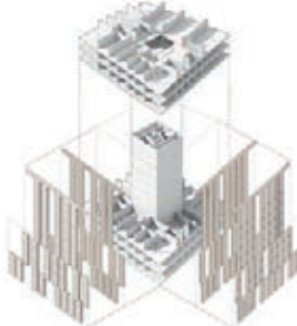
Explosionsschema Fassadenaufbau © Florian Krieger Architektur und Städtebau
