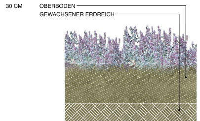
REGELDETAIL PFLANZFLÄCHE M 1:10
